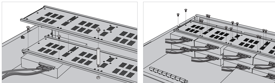
图3-2 安装硬盘
