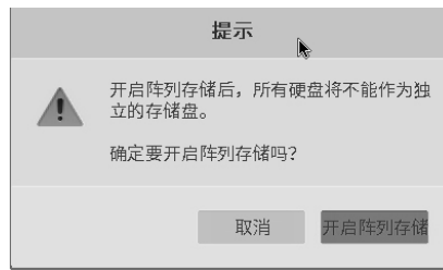
图4-12 确认风险
