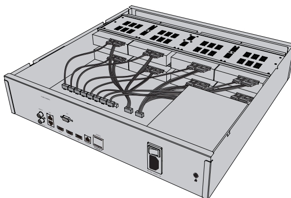
图3-3 完成安装
