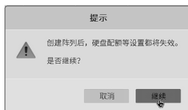
图4-14 确认创建
